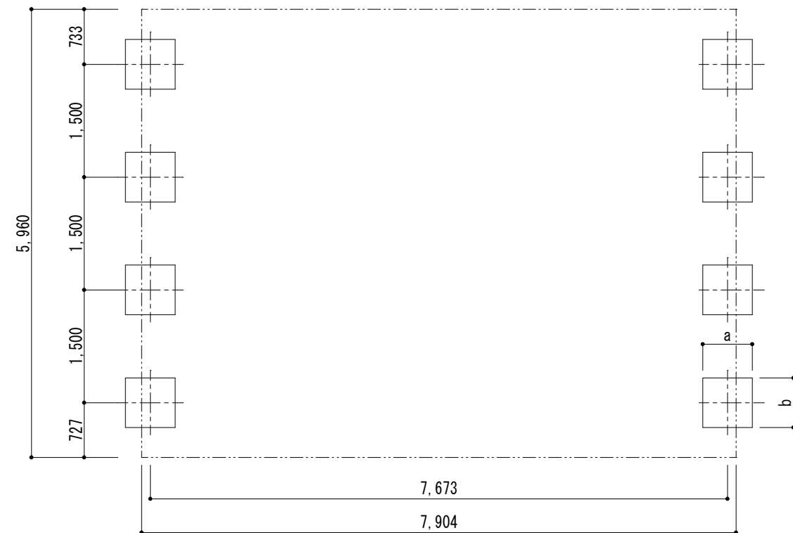
■ 基礎配置図
